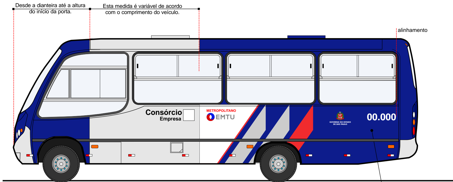
Vista lateral esquerda
