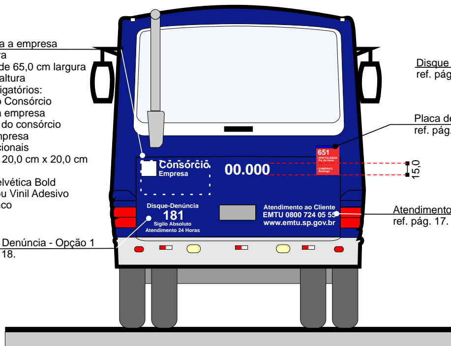
Vista traseira - Opção 1
